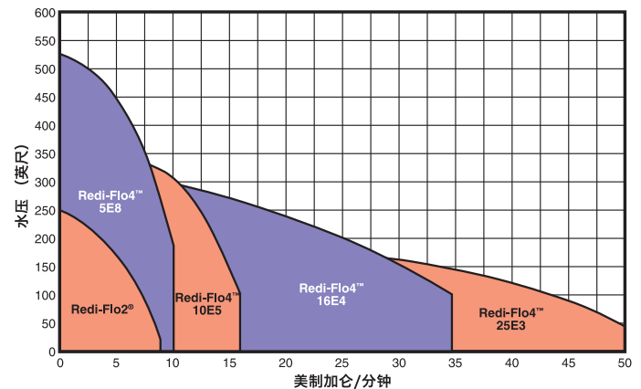
Redi-Flo2® and Redi-Flo4™变频泵工作曲线
